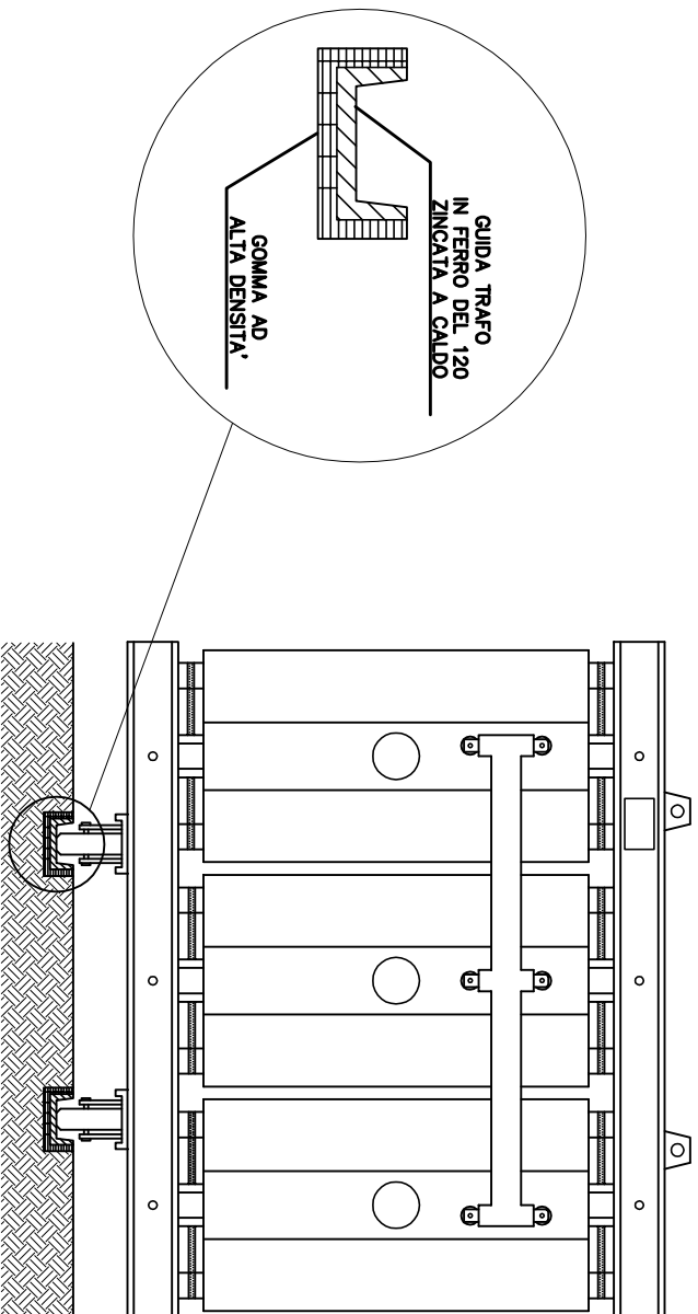
VISTA LATERALE
