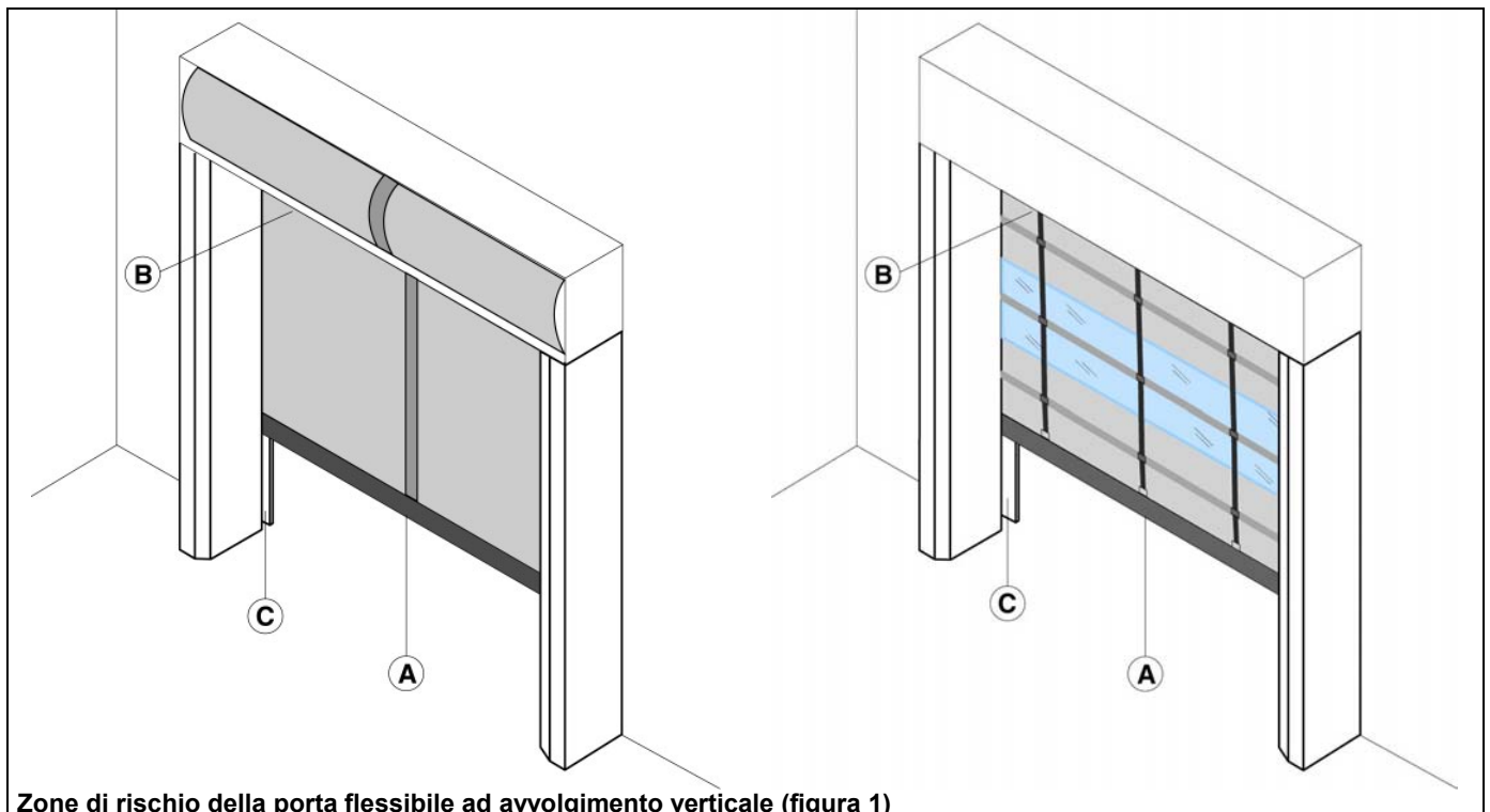
Zone di rischio della porta flessibile ad avvolgimento verticale (figura 1)
